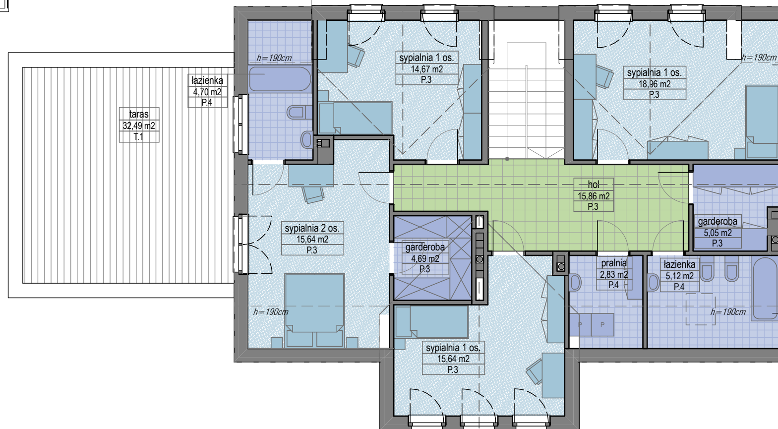
POZIOM +1
